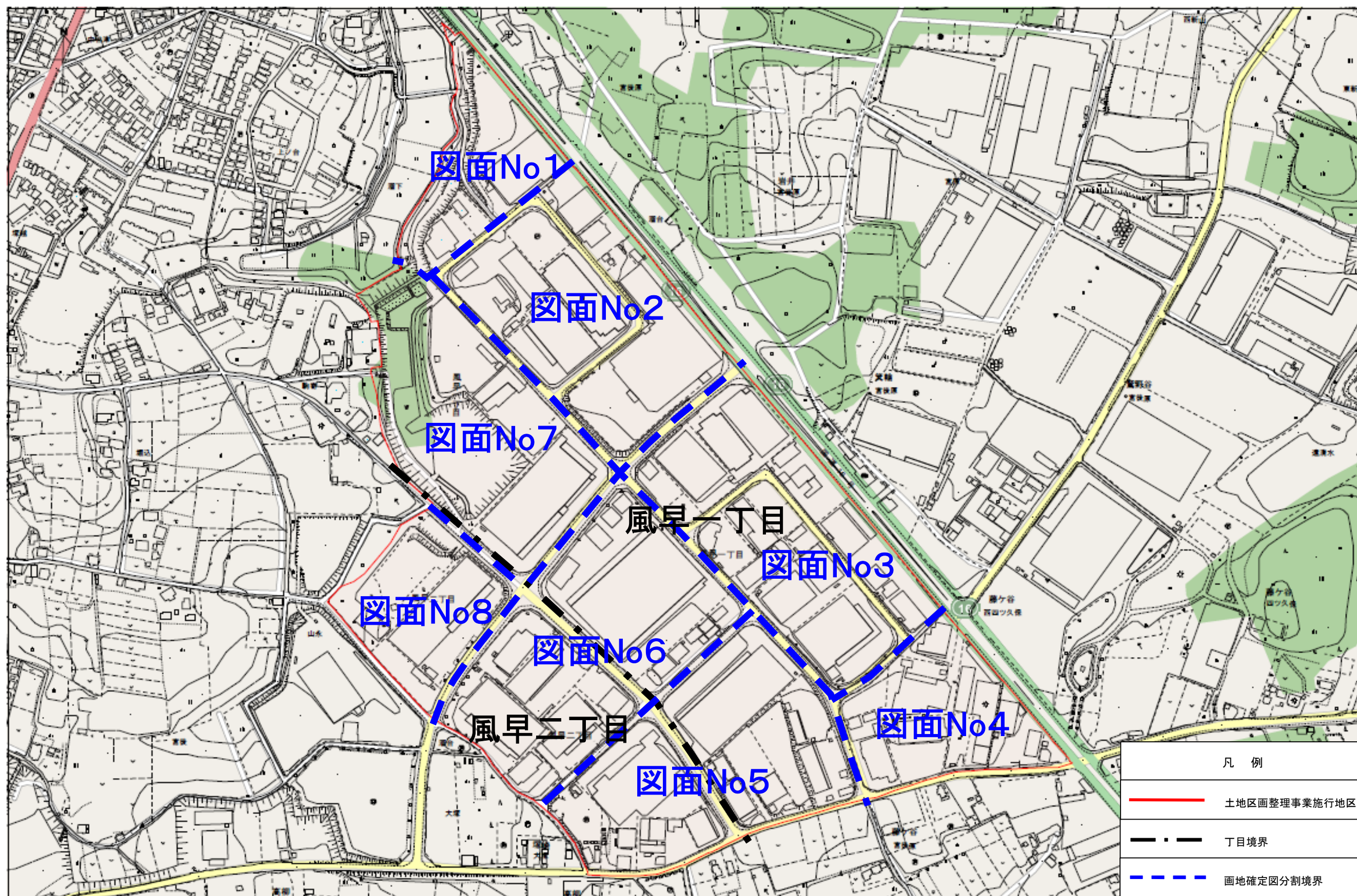
25 第二工業団地 画地出来形確認測量図 図郭割図
