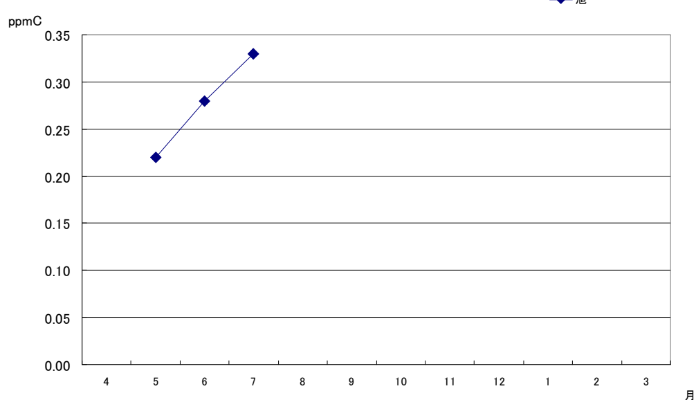
非メタン炭化水素の月平均値の月別変化（6～9時の3時間平均値）
