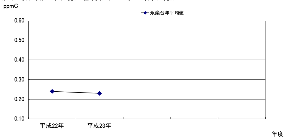
非メタン炭化水素の年平均値の経年変化(6～9時の3時間平均値)
