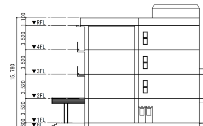
東立面图
