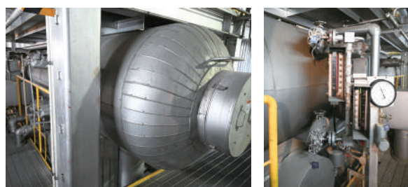
南部クリーンセンターのボイラの外観。焼却炉で発生する廃ガスの温度を下げると同時に、回収した熱で蒸気を生産させます
