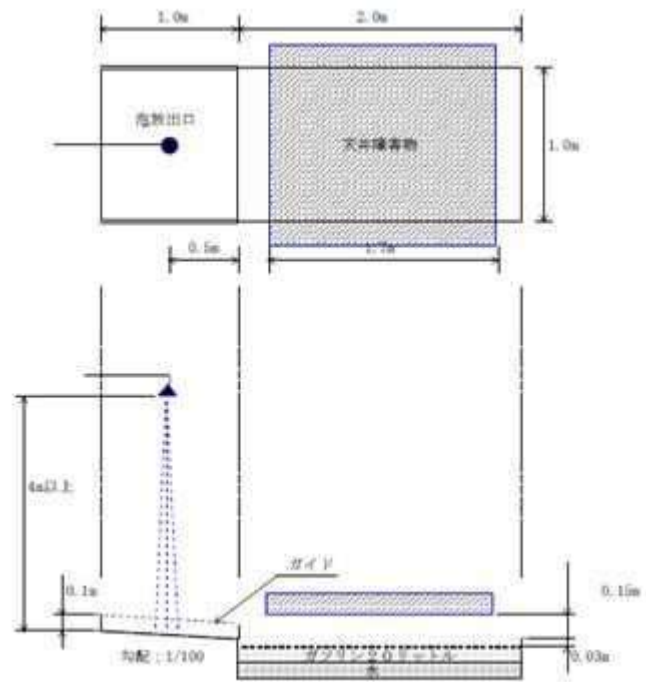
図 2 下方放出方式
