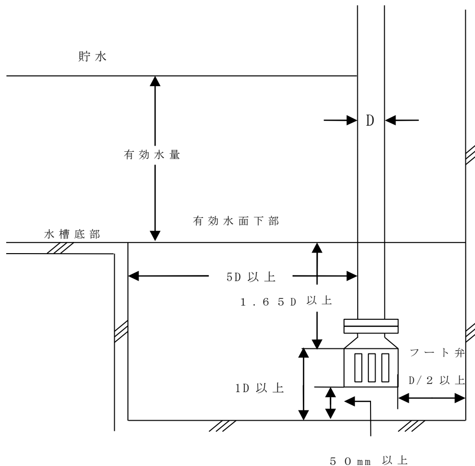
図 2 (サクシヨンピットを設ける場合)
