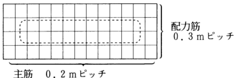
タンクふたの配筋例
