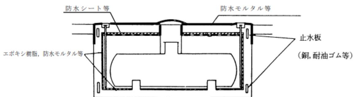
タンク室の防水措置の例
