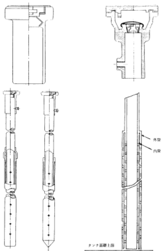
漏えい検査管の管体構造例
