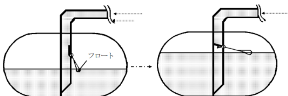
例図2 フロート方式
