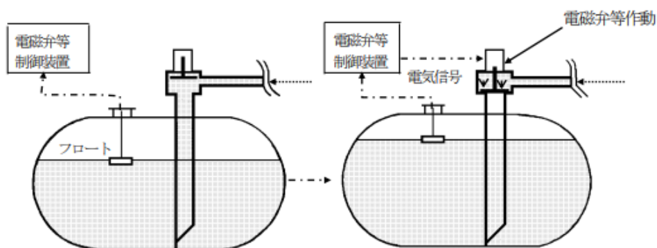
例図3 液面計連動型遮断方式
