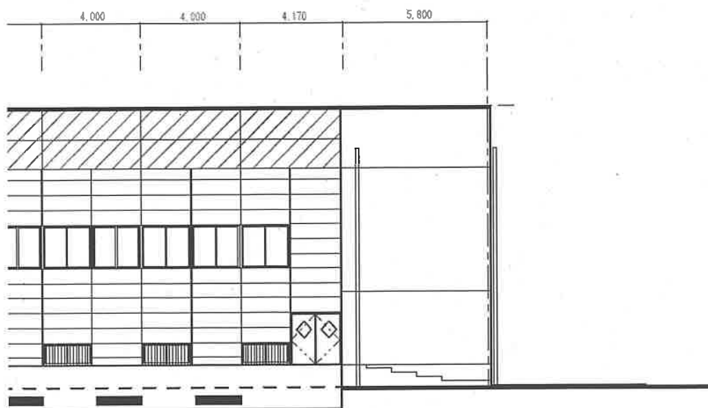
東立面図
