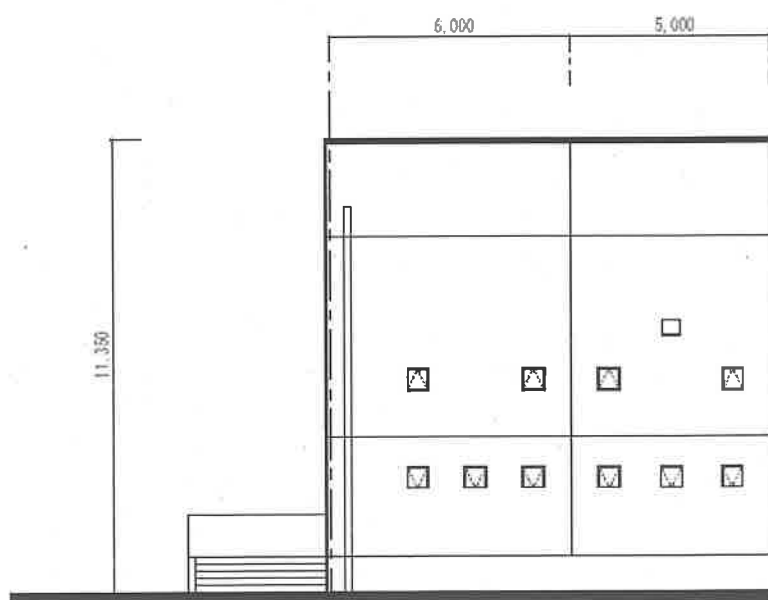
西立面图
