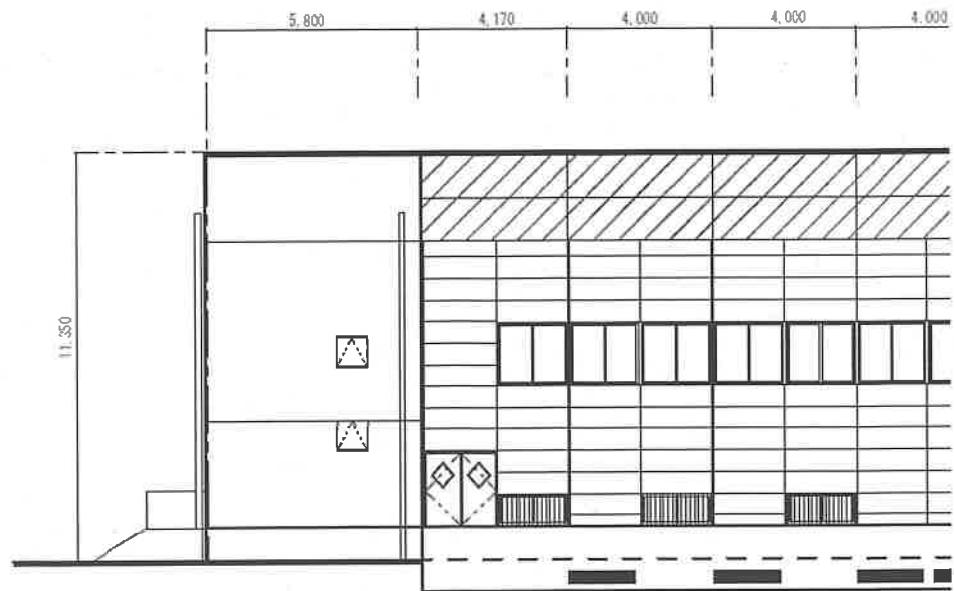
東立面图
