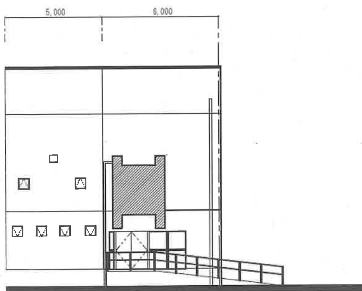
西立面图
