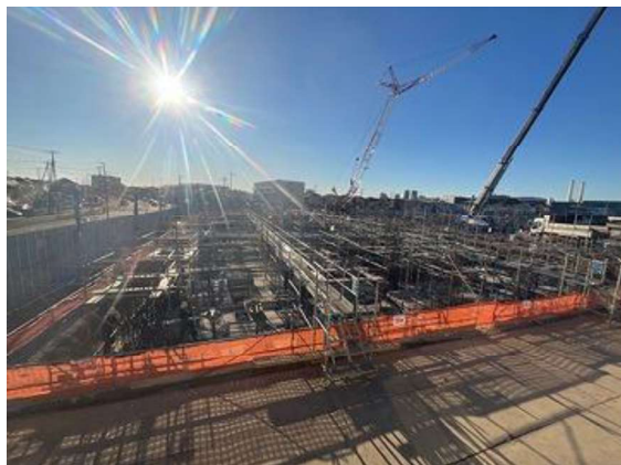
鉄筋工事（配筋状況）
