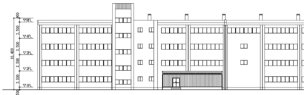
北立面图
