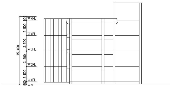
東立面图
