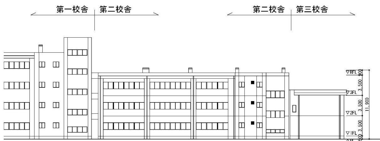
北立面图
