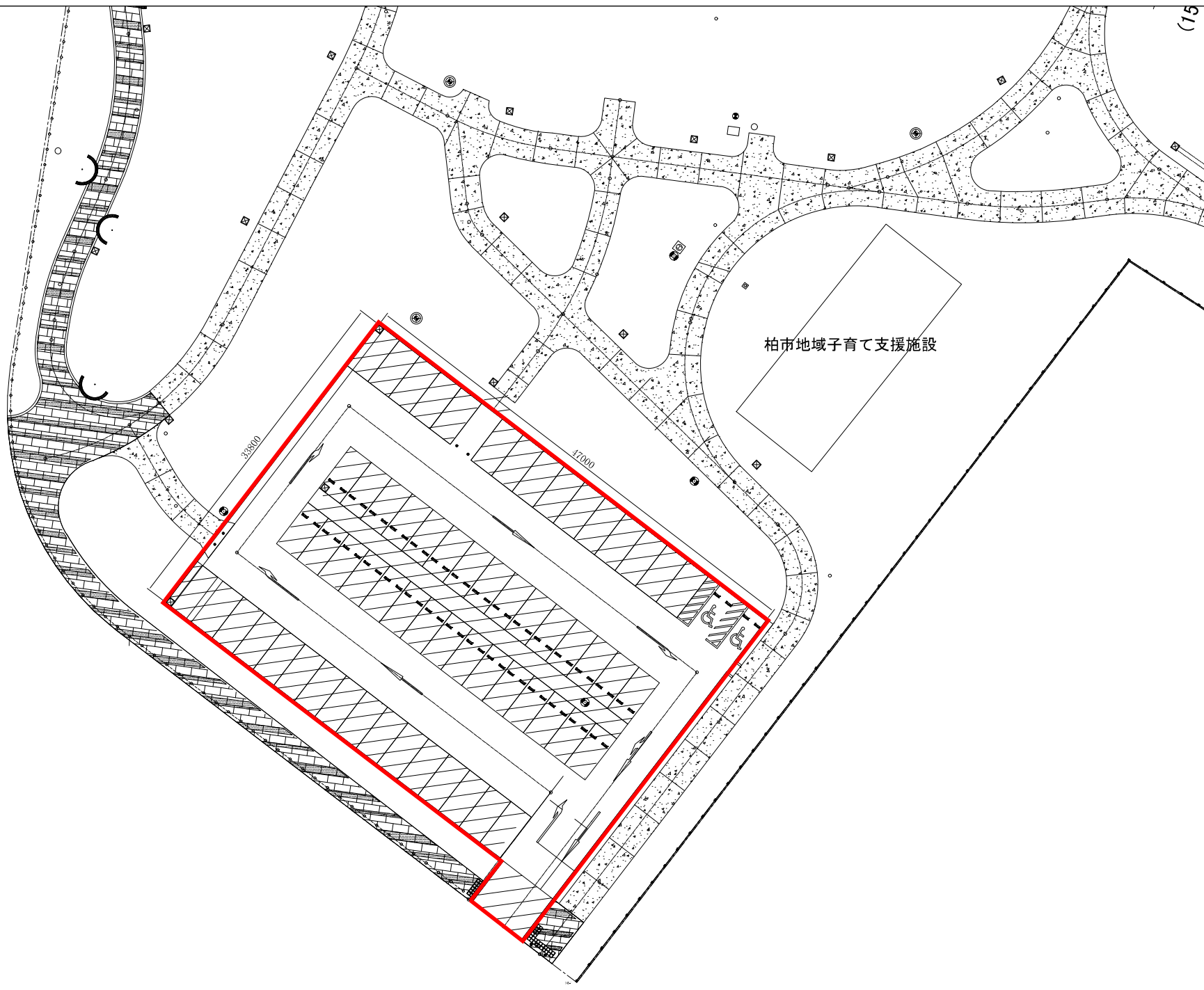
駐車場平面図 S=FREE
