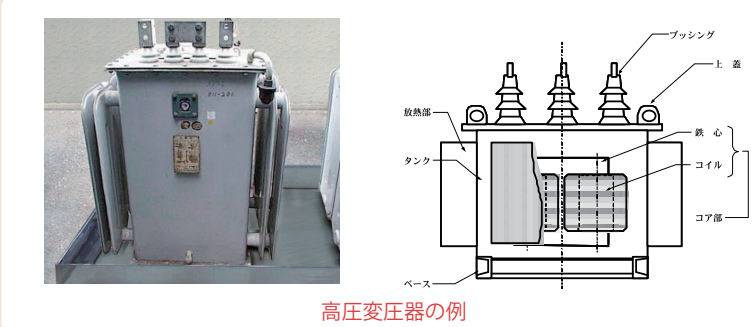
高圧変圧器の例
