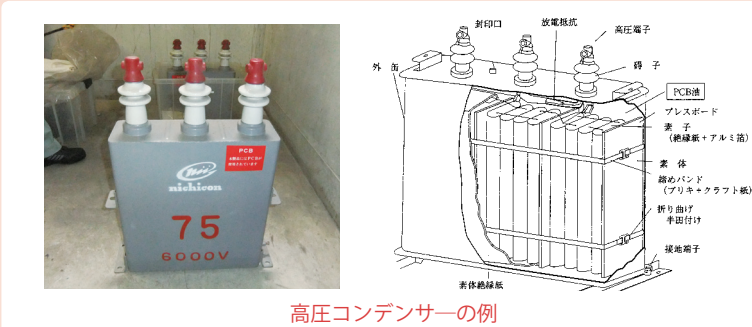
高圧コンデンサーの例
