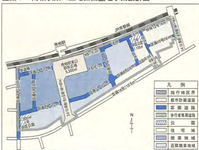
■図1 南柏駅東口土地区画整理事業設計図
