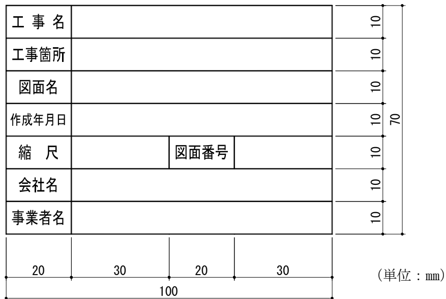
図- 2.1 表題欄の寸法及び様式
