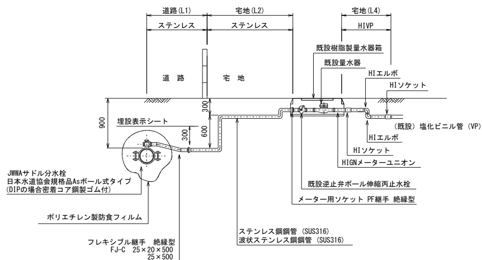
図- 3.13 給水管取直し工事 (A タイプ)
