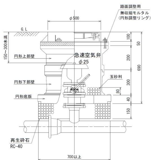
図- 3.31 空気弁断面図 (例) (単位：mm)
