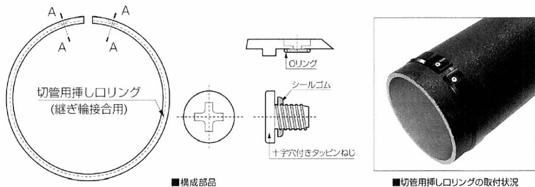
(参考) NS 形ダクトイル管 切管用挿しロリング
