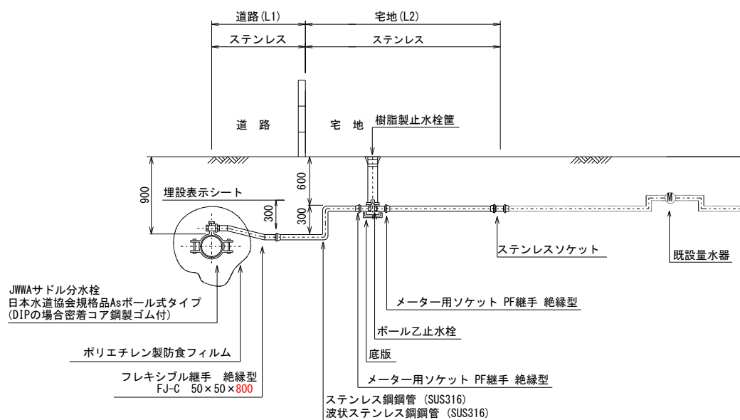
図- 3.15 給水管取直し工事 (B タイプ 50mm)
