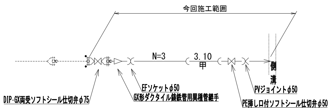
図-3.11 ダクトイル鋳鉄管からの延伸の場合
