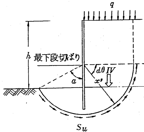
図-4 ヒービングの検討法
