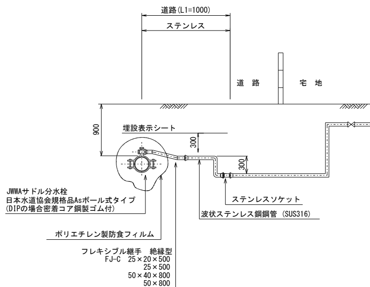
図- 3.16 給水管取直し工事 (C タイプ)
