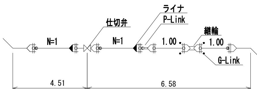
図- 3.8 耐震管路の寸法記入例 (GX φ100)
