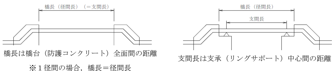
図 3-50 橋長・支間長のとり方
