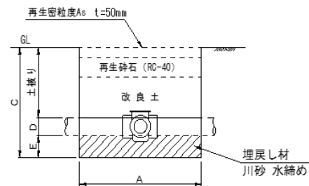
b-b' 断面図
