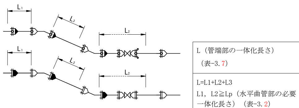
図- 3.5 既設管路との接続 (末端部)
