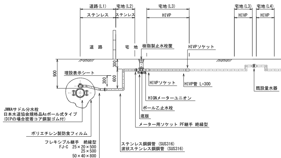
図-3.14 給水管取直し工事 (B タイプ)
