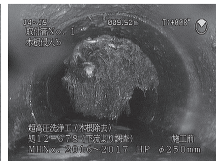
▲自走式カメラが捉えた下水道への取付管の突き出しや木の根の侵入の様子
