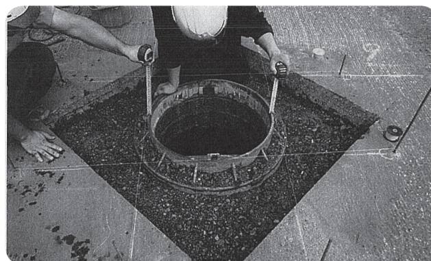
▲マンホール蓋を正確に設置するために、現状の大きさを確認しながら作業します
