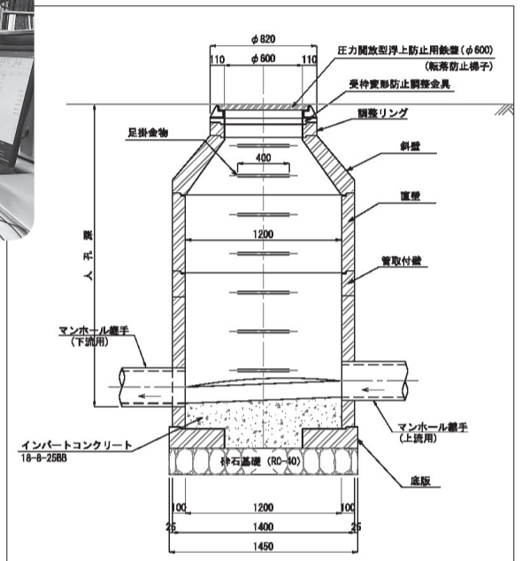
▲マンホールの断面図
